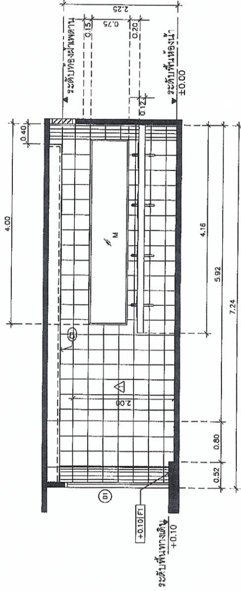
รูปด้าน 2 SCALE 1:50
