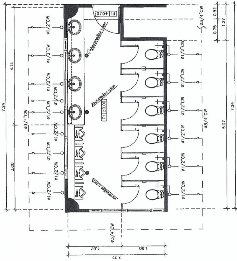
แปลนระบบท่อประปาห้องน้าย ชั้น 8
