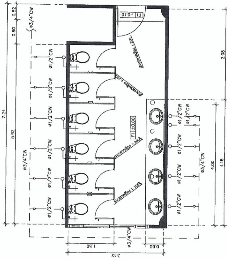
แปลนระบบท่อประปาห้องน้ำหญิง ชั้น 8
